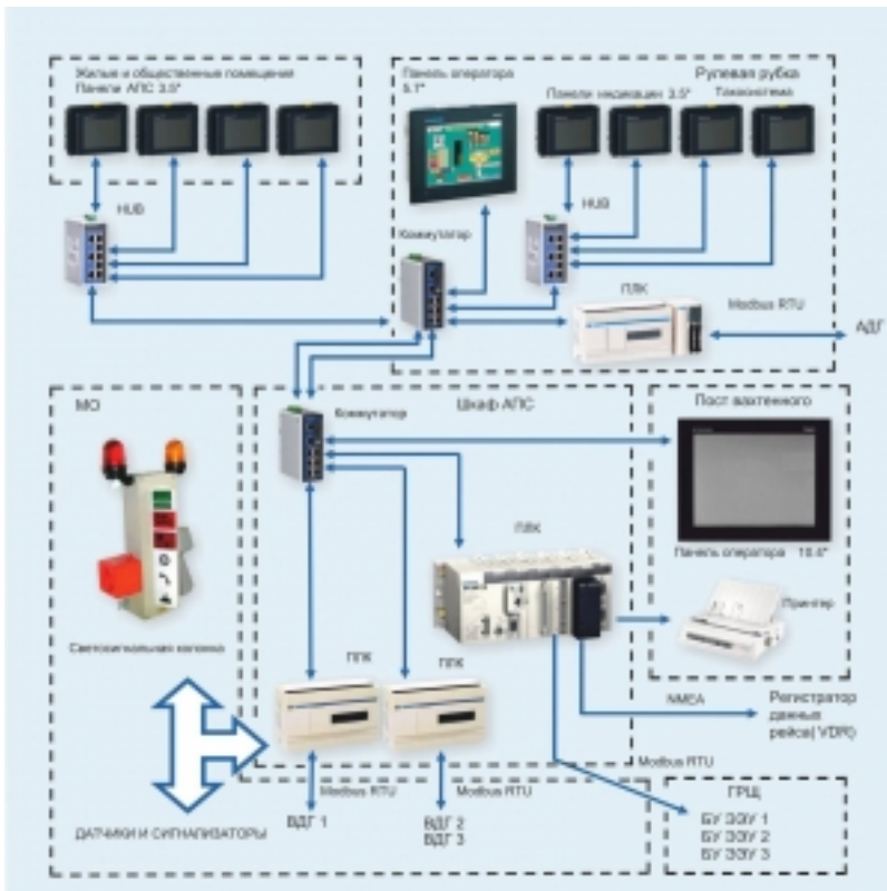
Наименование оборудования: Система аварийно-предупредительной сигнализации, индикации и защиты — «MANAGER 301M» Производитель: АКЦИОНЕРНОЕ ОБЩЕСТВО "МОРСКИЕ НАВИГАЦИОННЫЕ СИСТЕМЫ"
