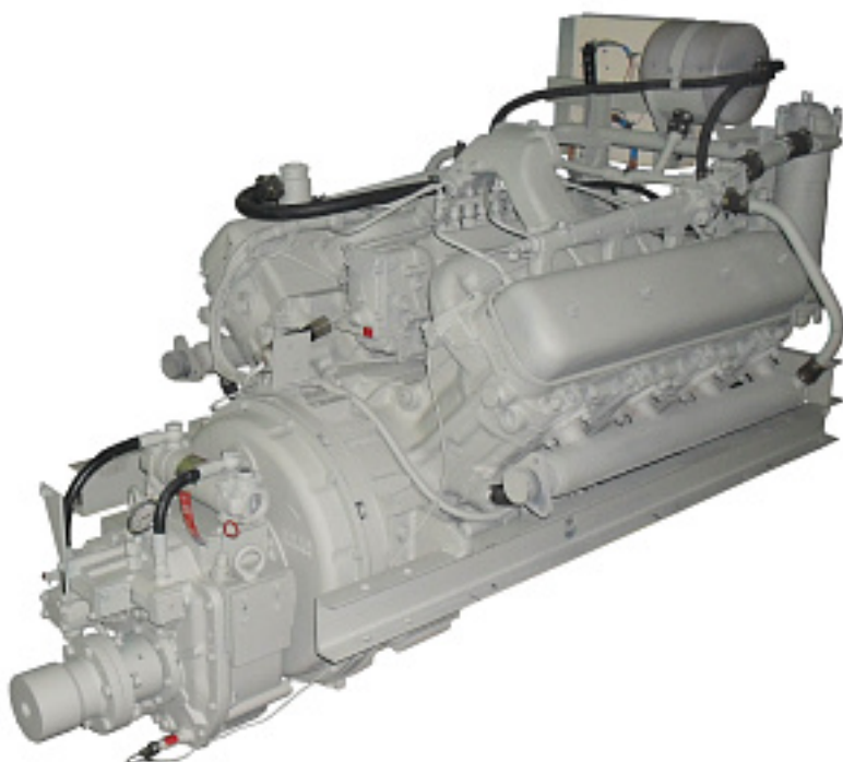
Наименование оборудования: ДРА 163-201/1500-2100 Производитель: ОБЩЕСТВО С ОГРАНИЧЕННОЙ ОТВЕТСТВЕННОСТЬЮ "АЛТАЙСКИЙ ЗАВОД ДИЗЕЛЬНЫХ АГРЕГАТОВ"
