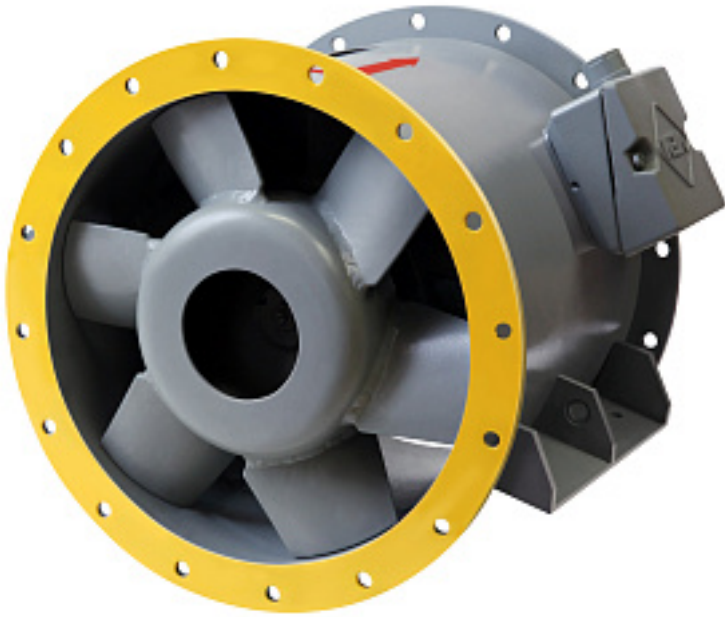
Наименование оборудования: Электровентилятор судовой осевой ВОС 360/20 Производитель: ОБЩЕСТВО С ОГРАНИЧЕННОЙ ОТВЕТСТВЕННОСТЬЮ "ИННОВЕНТ"
