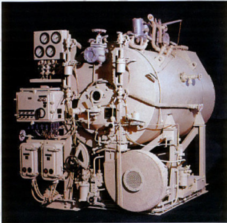
Наименование оборудования: Котлоагрегат паровой КОАВ-63 Производитель: ОБЩЕСТВО С ОГРАНИЧЕННОЙ ОТВЕТСТВЕННОСТЬЮ "СТМ-ОСКОЛ"
