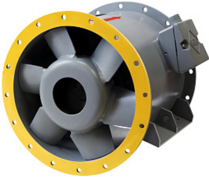
Наименование оборудования: Электровентилятор судовой осевой ВОС 10/2 Производитель: ОБЩЕСТВО С ОГРАНИЧЕННОЙ ОТВЕТСТВЕННОСТЬЮ "ИННОВЕНТ"
