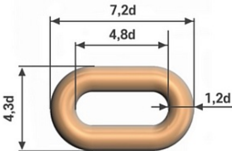
Наименование оборудования: Звено концевое (комплектующие якорной цепи) Производитель: ПУБЛИЧНОЕ АКЦИОНЕРНОЕ ОБЩЕСТВО "ЗАВОД КРАСНЫЙ ЯКОРЬ"
