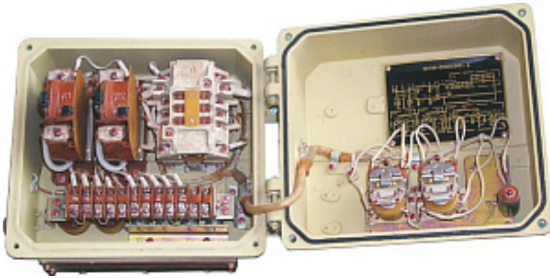
Наименование оборудования: Пускатели магнитные серии ПМТМ-01000-Д Производитель: ОТКРЫТОЕ АКЦИОНЕРНОЕ ОБЩЕСТВО "МЕДНОГОРСКИЙ ЭЛЕКТРОТЕХНИЧЕСКИЙ ЗАВОД "УРАЛЭЛЕКТРО"
