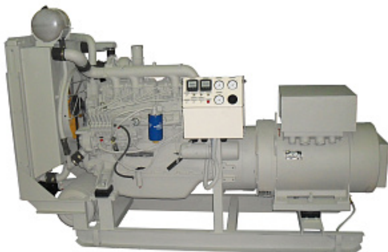
Наименование оборудования: ДГ75(Р)-1/2А.А/В-230/400 Производитель: ОБЩЕСТВО С ОГРАНИЧЕННОЙ ОТВЕТСТВЕННОСТЬЮ "АЛТАЙСКИЙ ЗАВОД ДИЗЕЛЬНЫХ АГРЕГАТОВ"
