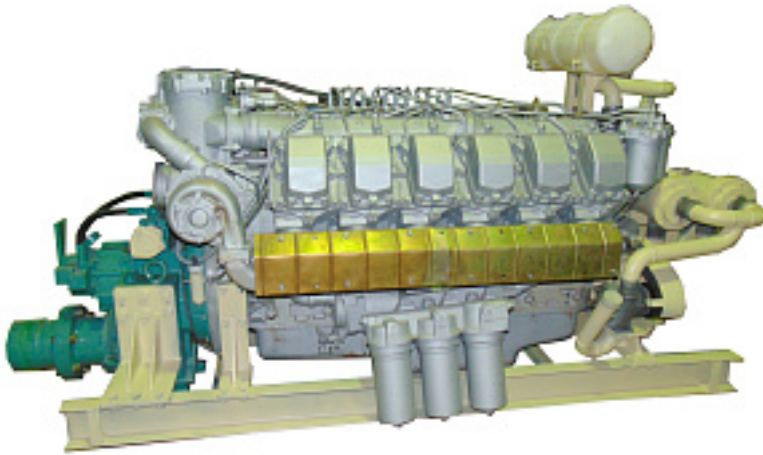
Наименование оборудования: ДРА 405-600/1500-2100 Производитель: ОБЩЕСТВО С ОГРАНИЧЕННОЙ ОТВЕТСТВЕННОСТЬЮ "АЛТАЙСКИЙ ЗАВОД ДИЗЕЛЬНЫХ АГРЕГАТОВ"
