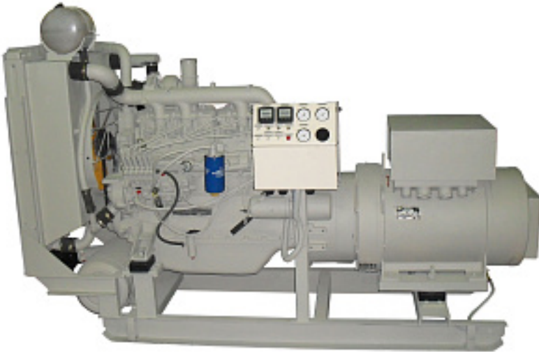
Наименование оборудования: ДГ50(Р)-1/2А.А/Р/В-230/400 Производитель: ОБЩЕСТВО С ОГРАНИЧЕННОЙ ОТВЕТСТВЕННОСТЬЮ "АЛТАЙСКИЙ ЗАВОД ДИЗЕЛЬНЫХ АГРЕГАТОВ"
