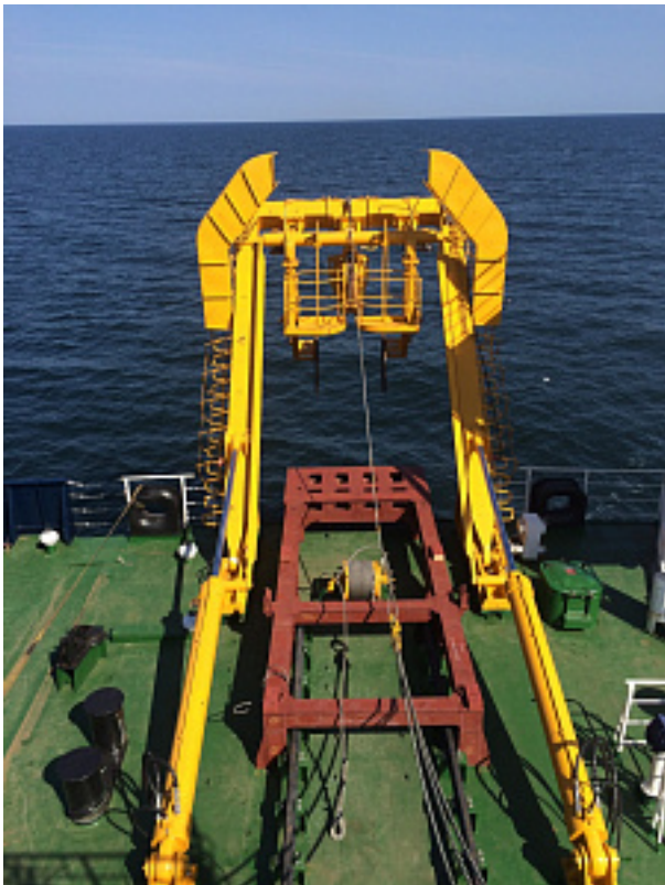
Наименование оборудования: Кормовое спуско-подъемное и буксирное устройство КСПУ Производитель: АКЦИОНЕРНОЕ ОБЩЕСТВО "ОБУХОВСКОЕ"
