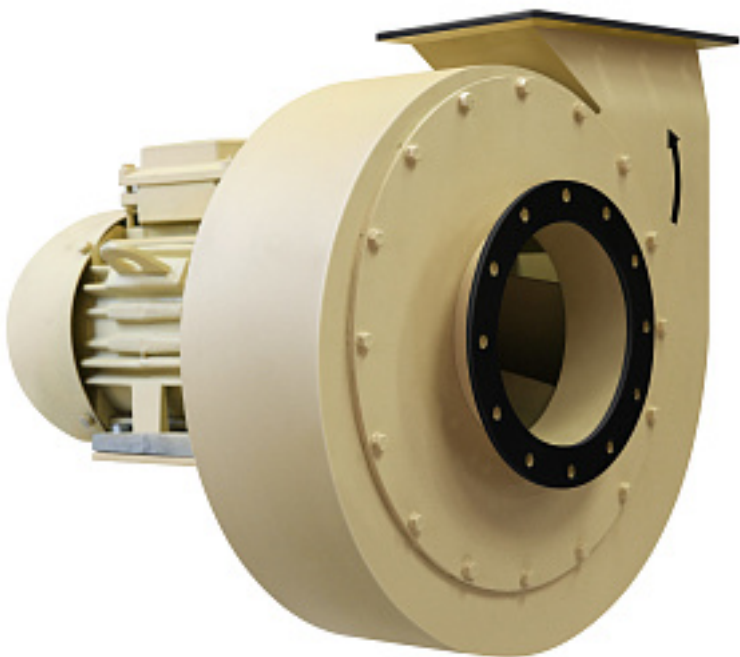
Наименование оборудования: Электровентиль радиальный судовой РСС 2,5/10 Производитель: ОБЩЕСТВО С ОГРАНИЧЕННОЙ ОТВЕТСТВЕННОСТЬЮ "ИННОВЕНТ"
