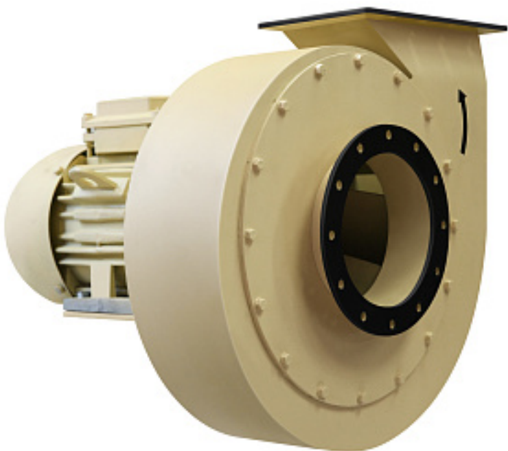
Наименование оборудования: Электровентиль радиальный судовой РСС 25/16 Производитель: ОБЩЕСТВО С ОГРАНИЧЕННОЙ ОТВЕТСТВЕННОСТЬЮ "ИННОВЕНТ"
