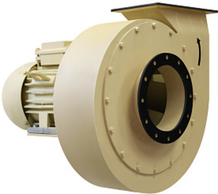
Наименование оборудования: Электровентиль радиальный судовой РСС 16/16 Производитель: ОБЩЕСТВО С ОГРАНИЧЕННОЙ ОТВЕТСТВЕННОСТЬЮ "ИННОВЕНТ"
