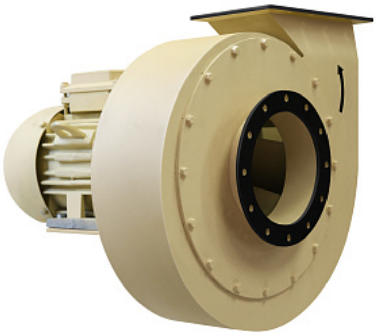
Наименование оборудования: Электровентиль радиальный судовой РСС 25/40 Производитель: ОБЩЕСТВО С ОГРАНИЧЕННОЙ ОТВЕТСТВЕННОСТЬЮ "ИННОВЕНТ"
