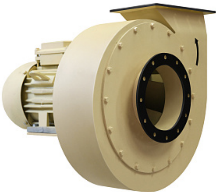
Наименование оборудования: Электровентиль радиальный судовой РСС 2,5/25 Производитель: ОБЩЕСТВО С ОГРАНИЧЕННОЙ ОТВЕТСТВЕННОСТЬЮ "ИННОВЕНТ"
