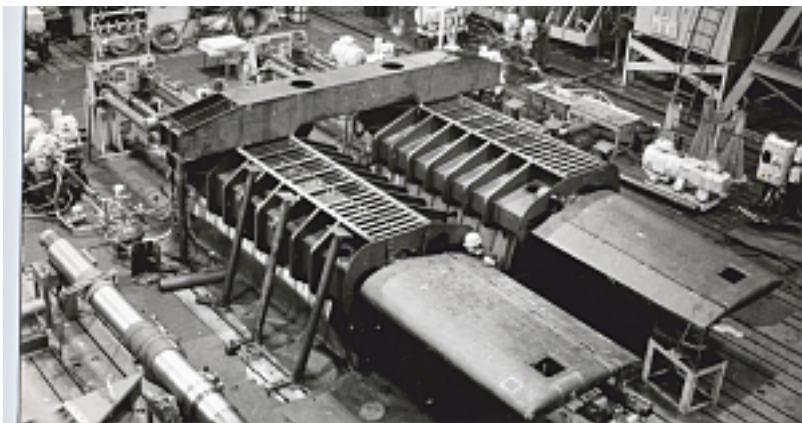
Наименование оборудования: Успокоитель качки с выдвижными рулями УК-134-5 Производитель: ЗАКРЫТОЕ АКЦИОНЕРНОЕ ОБЩЕСТВО "ЦЕНТРАЛЬНЫЙ НАУЧНО-ИССЛЕДОВАТЕЛЬСКИЙ ИНСТИТУТ СУДОВОГО МАШИНОСТРОЕНИЯ"
