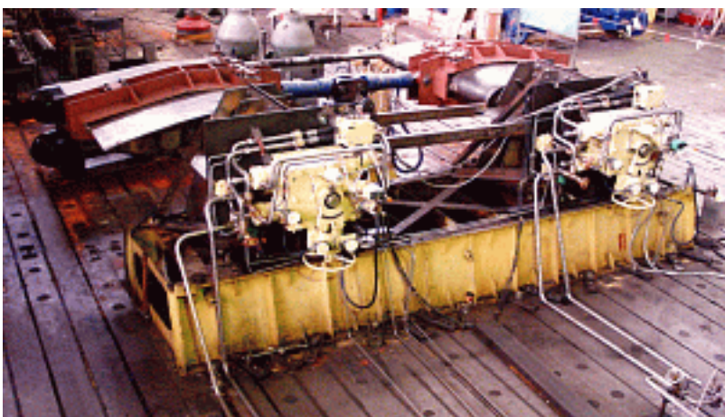
Наименование оборудования: Успокоители качки с неубирающимися рулями УК6-1 Производитель: ЗАКРЫТОЕ АКЦИОНЕРНОЕ ОБЩЕСТВО "ЦЕНТРАЛЬНЫЙ НАУЧНО-ИССЛЕДОВАТЕЛЬСКИЙ ИНСТИТУТ СУДОВОГО МАШИНОСТРОЕНИЯ"
