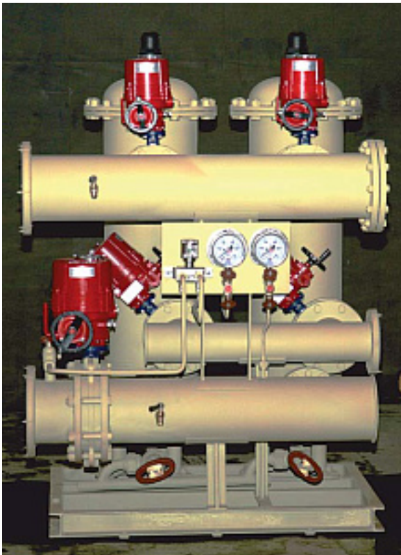
Наименование оборудования: Установка фильтрации морской воды СООБ-Ф 250 Производитель: ЗАКРЫТОЕ АКЦИОНЕРНОЕ ОБЩЕСТВО "ЦЕНТРАЛЬНЫЙ НАУЧНО-ИССЛЕДОВАТЕЛЬСКИЙ ИНСТИТУТ СУДОВОГО МАШИНОСТРОЕНИЯ"
