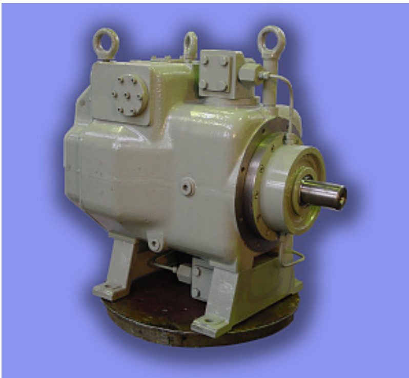
Наименование оборудования: Насосы аксиально-поршневые регулируемые НК 40 Производитель: ЗАКРЫТОЕ АКЦИОНЕРНОЕ ОБЩЕСТВО "ЦЕНТРАЛЬНЫЙ НАУЧНО-ИССЛЕДОВАТЕЛЬСКИЙ ИНСТИТУТ СУДОВОГО МАШИНОСТРОЕНИЯ"
