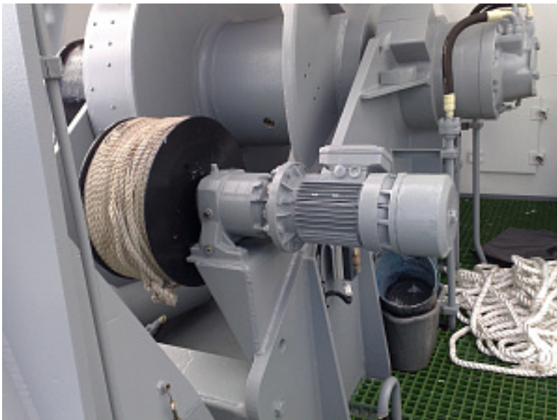
Наименование оборудования: Шпиль якорно-швартовый Производитель: ОБЩЕСТВО С ОГРАНИЧЕННОЙ ОТВЕТСТВЕННОСТЬЮ "СУДОСТРОЕНИЕ СУДОРЕМОНТ"
