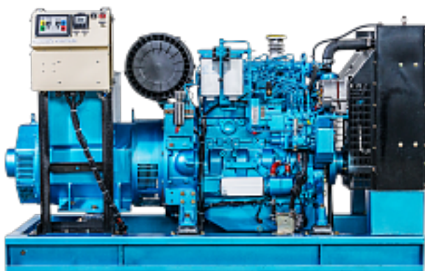
Наименование оборудования: АДГР-24/1500 серии РД 1000 Производитель: ОБЩЕСТВО С ОГРАНИЧЕННОЙ ОТВЕТСТВЕННОСТЬЮ "ЗАВОД СУДОВЫХ ДВИГАТЕЛЕЙ "РЕМДИЗЕЛЬ"
