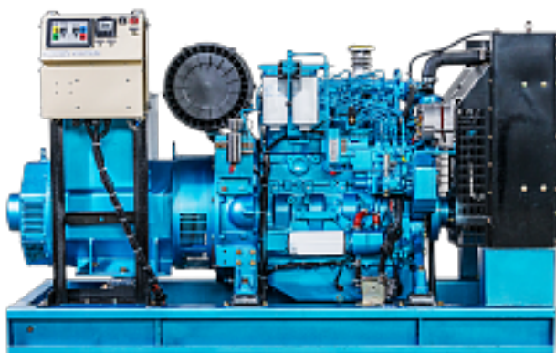
Наименование оборудования: АДГР-150/1500 серии РД 1000 Производитель: ОБЩЕСТВО С ОГРАНИЧЕННОЙ ОТВЕТСТВЕННОСТЬЮ "ЗАВОД СУДОВЫХ ДВИГАТЕЛЕЙ "РЕМДИЗЕЛЬ"
